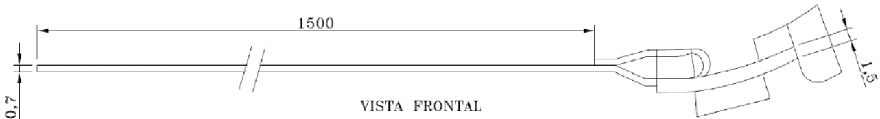
Figura 2 - Fita em aço inoxidável (item 5)
