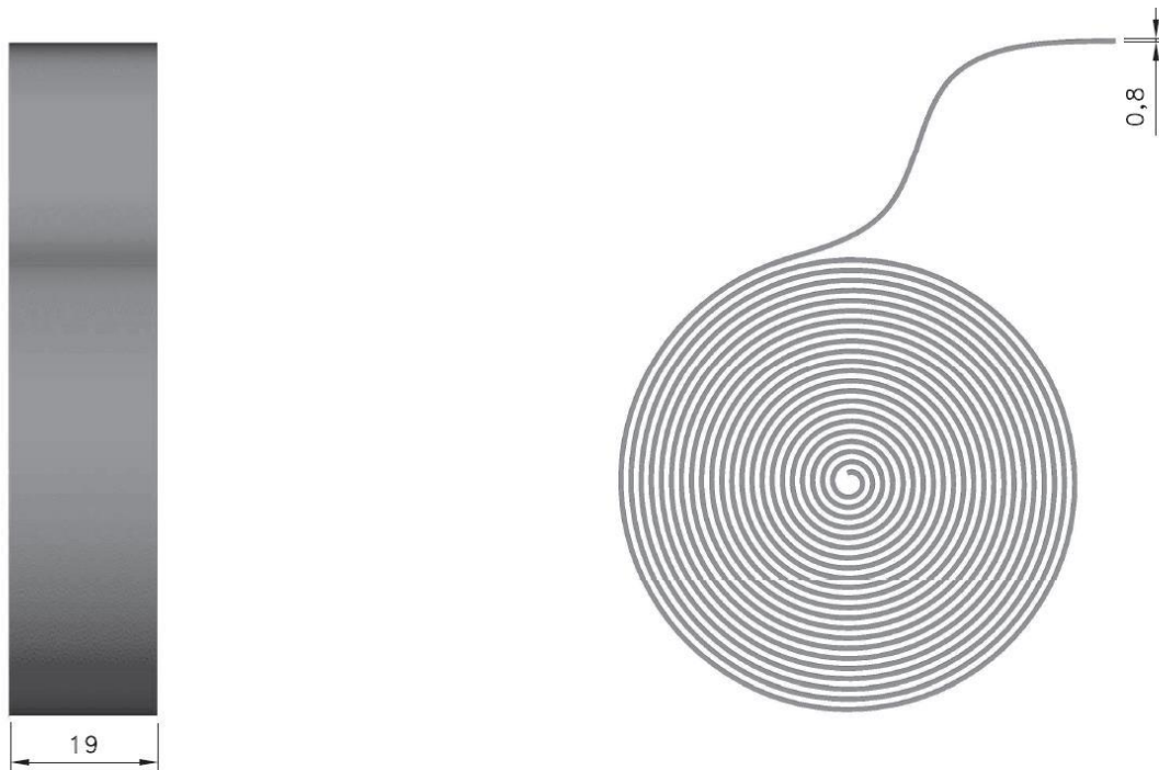
VISTA LATERAL ESQUERDA
